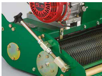
Ajuste de altura de operación sencilla y sin herramientas
