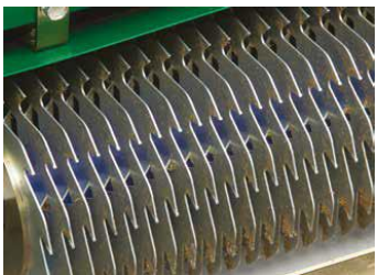
El último cortador de verti-cutter con cuchillas con punta de tungsteno
