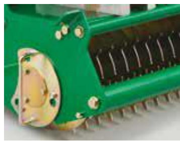
Bloqueo de carrete de cambio simple
